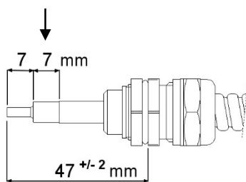
Figura 7: acabado del cable de alta tensión azul
