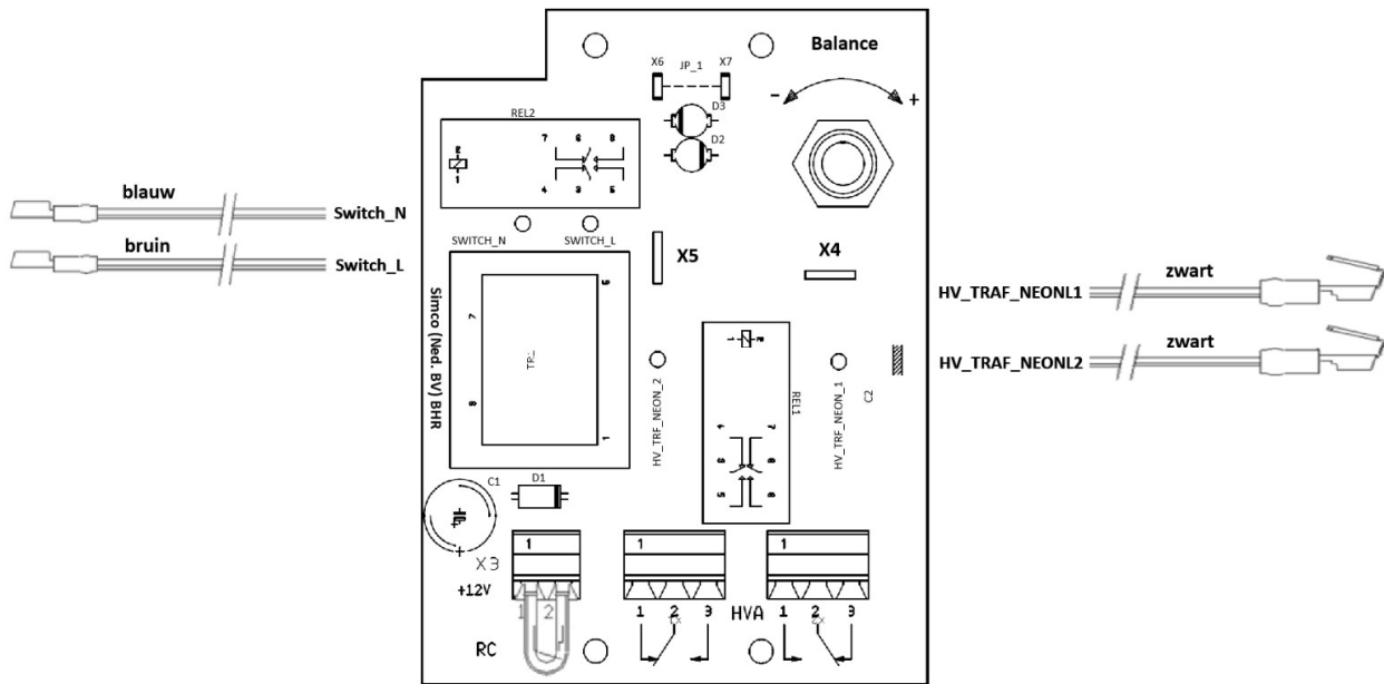
Figura 10: Placa de circuito impreso BHR opcional
