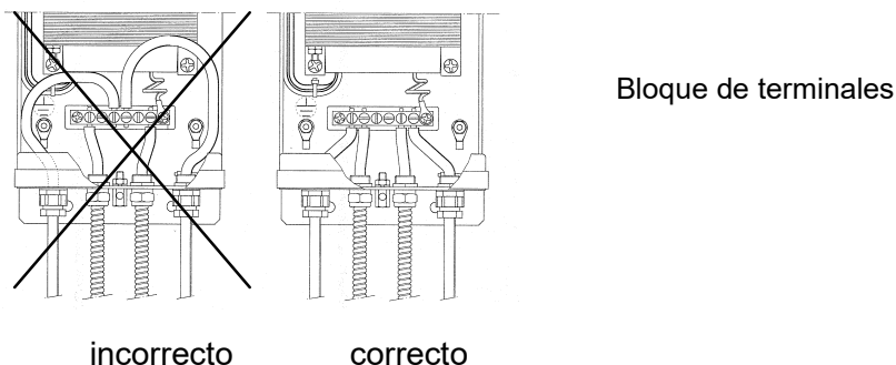
Figura 3: Conexión del cable en la unidad de alimentación
