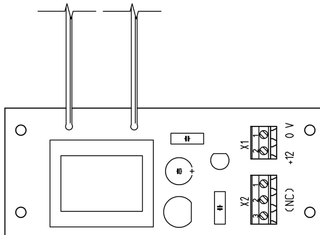
Figura 12: Circuito stampato opzionale M
