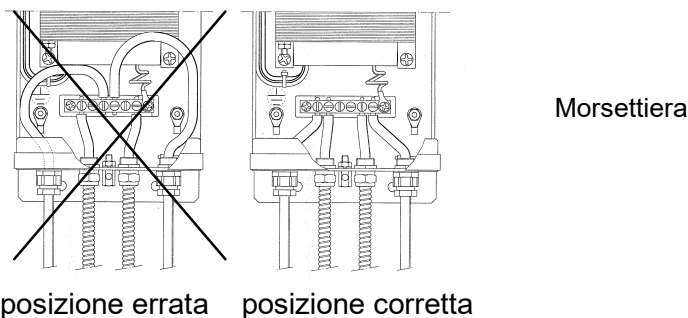
Figura 3: Collegamento del cavo nell'unità di alimentazione
