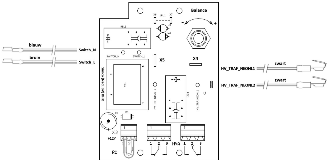
Figura 10: Circuito stampato opzionale BHR
